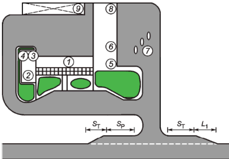
Рисунок А.10 - Пример (схема) размещения пассажирской автостанции вместимостью 50 человек
