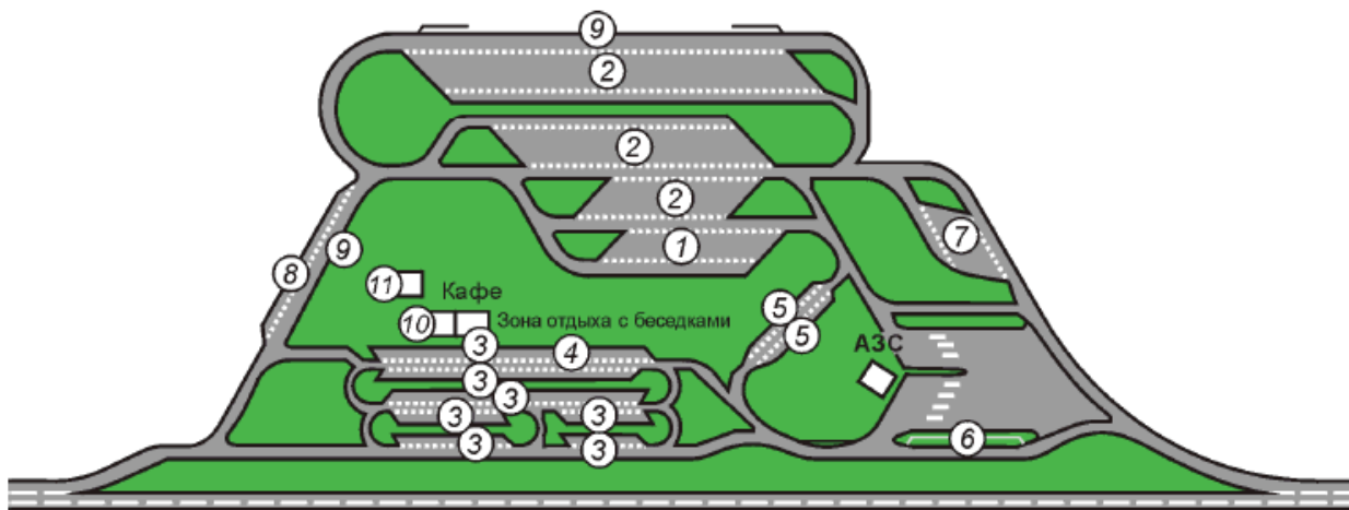
Рисунок А.4 - Вариант 4 размещения автозаправочной станции совместно с кафе и площадкой отдыха
