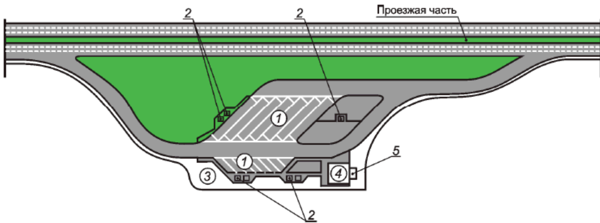
Рисунок А.6 - Пример (схема) размещения большой площадки отдыха
